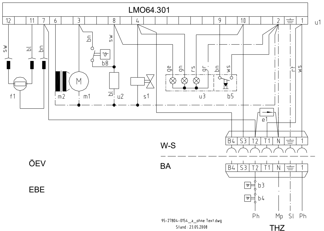
Abb. 14: Schaltplan mit Gebläsenachlauf für RE 1 HG
