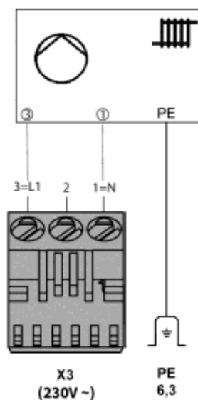
Abb. 24: Anschluss externe Heizkreispumpe
