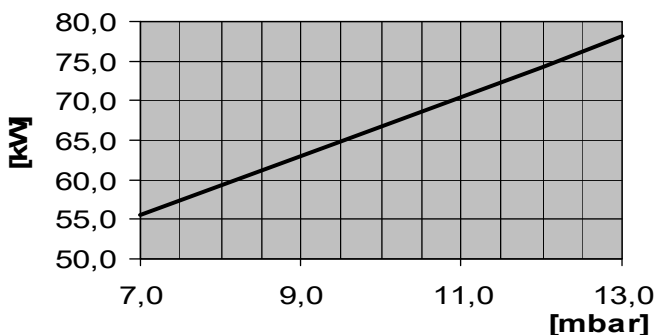
Abb. 22: Leistungsdiagramm RE 1.70 H
