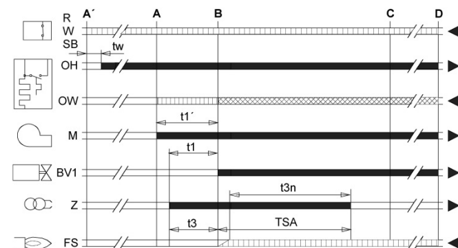
Abb. 27: Programmablauf LMO 14.155
