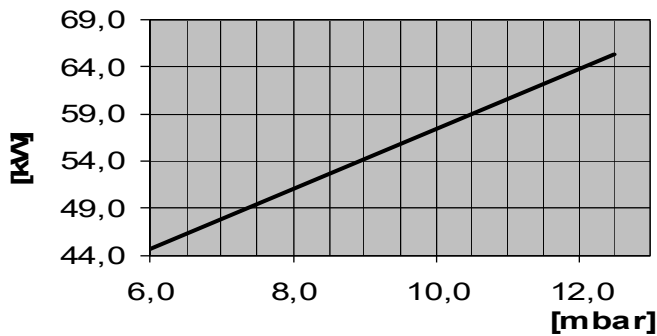
Abb. 21: Leistungsdiagramm RE 1.60 H
