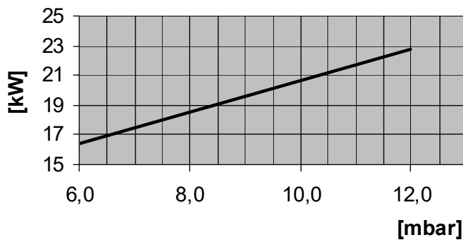
Abb. 15: Leistungsdiagramm RE 1.22 H
