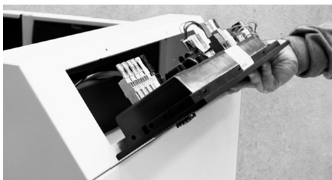
Abb. 18: Ausgeklapptes Unit-Schaltfeld
