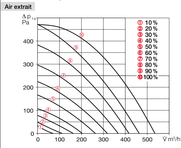
Courbe caractéristique KWL 500 W
