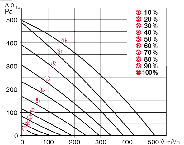
Kennlinie KWL 500 W ET
