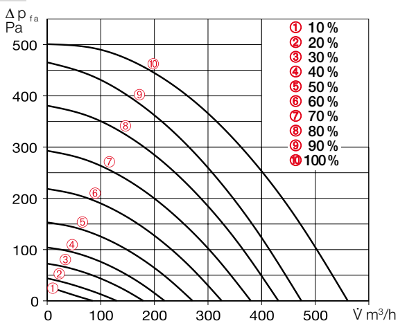
Kennlinie KWL 500 W ET
