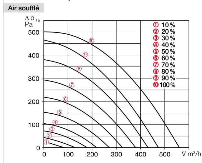
Courbe caractéristique KWL 500 W ET
