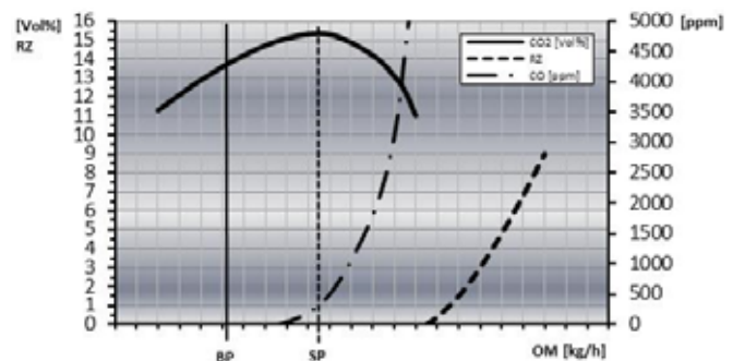
Abb. 51: Änderung der Heizölmenge bei konstanter Luftmenge
