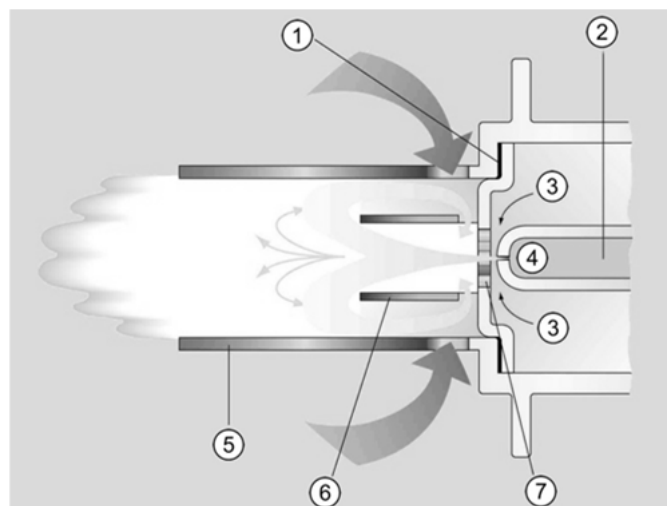
Abb. 52: Verbrennungsablauf Raketenbrenne®
