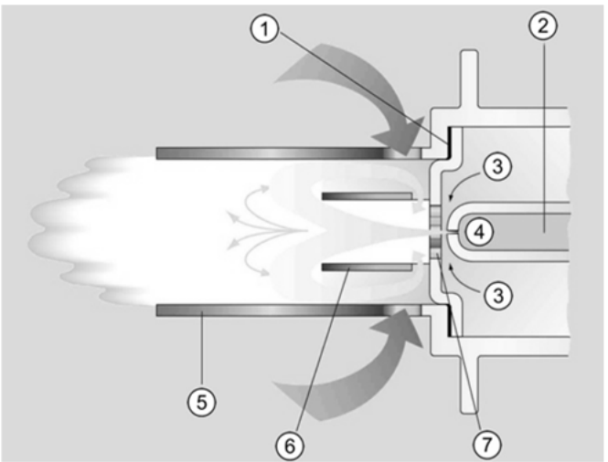
Abb. 52: Verbrennungsablauf Raketenbrenner®
