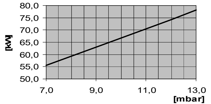
Abb. 26: Leistungsdiagramm RE 1.70 H
