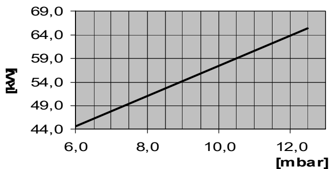
Abb. 25: Leistungsdiagramm RE 1.60 H
