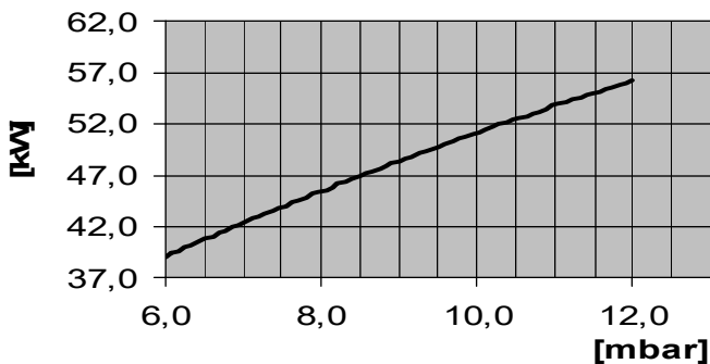
Abb. 24: Leistungsdiagramm RE 1.50 H
