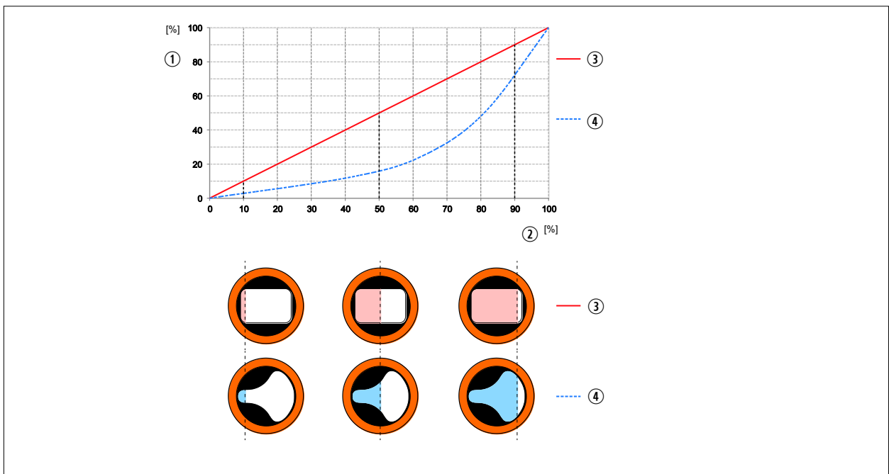
Abb. 6.6 progressive Kennlinie / Mischerverhalten
