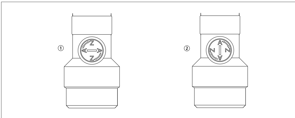
Abb. 8.3 Schwerkraftbremse
