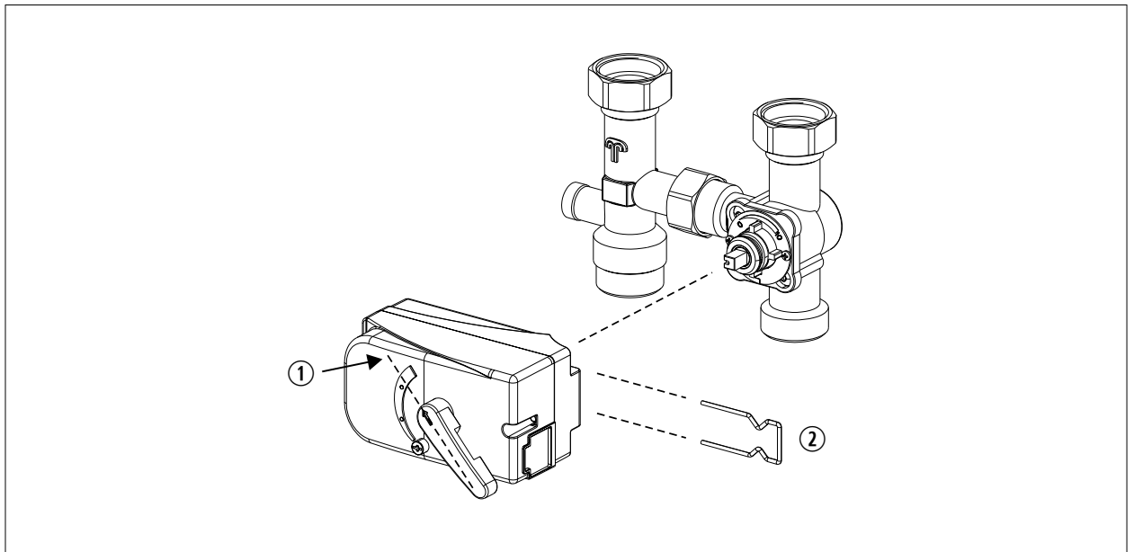
Abb. 6.3 Stellmotor demontieren
