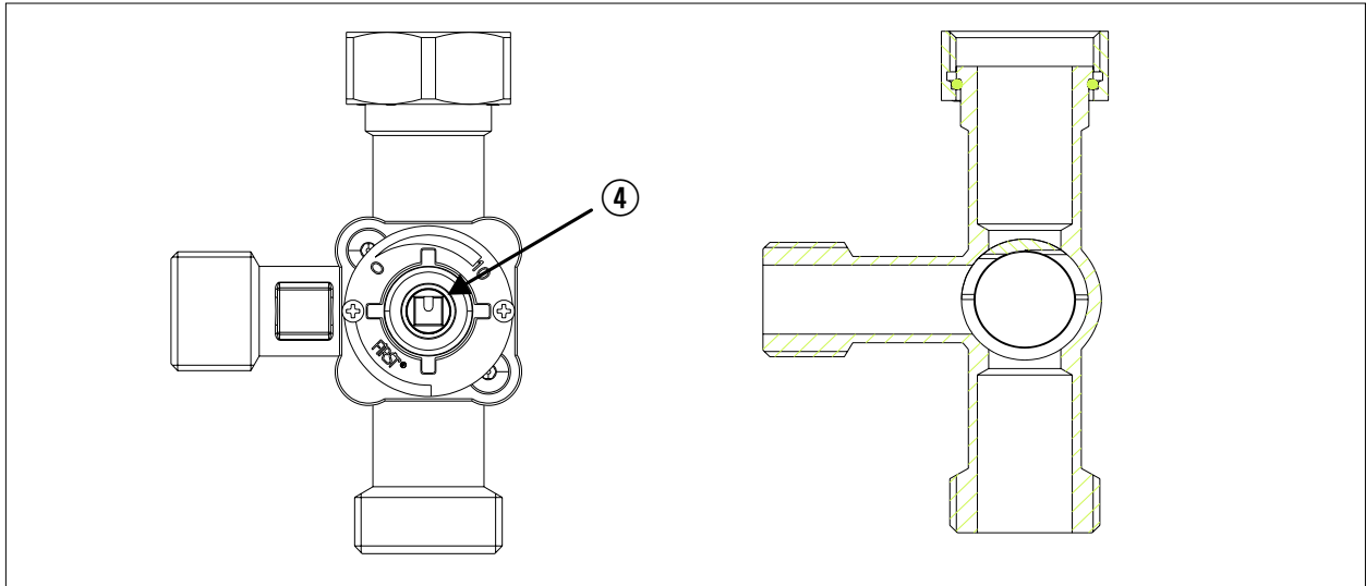
Abb. 6.5 Drehschieber
