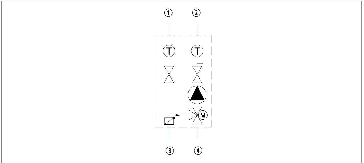
Abb. 6.7 Hydraulischer Anschluss
