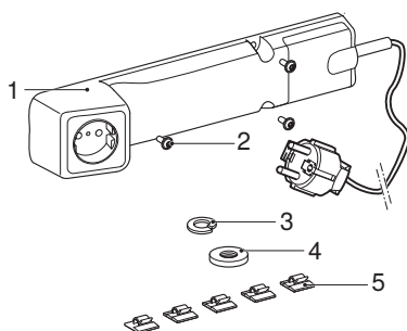
Bild 1: Geberit eluttagselement
