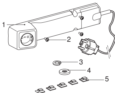
Kuva 1: Geberit-pistorasia
