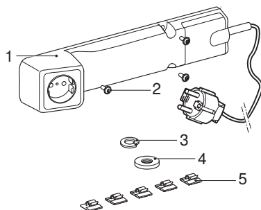
Slika 1: Element z vtičnico Geberit
