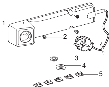
Figura 1: Elemento presa elettrica Geberit
