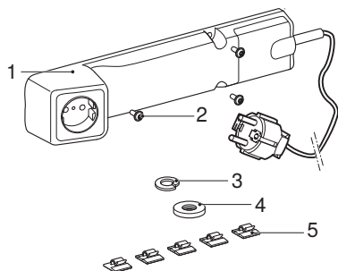
Abbildung 1: Geberit Steckdosenelement
