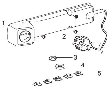
Joonis 1: Geberiti pistikupesa element
