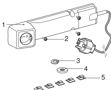
Obrázek 1: Prvek síťové zásuvky Geberit
