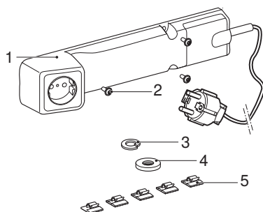
Фигура 1: Елемент за контакт Geberit
