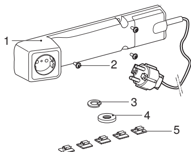
Рисунок 1: Розеточный модуль Geberit
