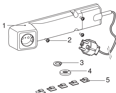
Bilde 1: Geberit stikkontaktelement
