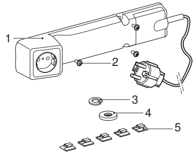
1 الشكل: عنصر مقبس Geberit
