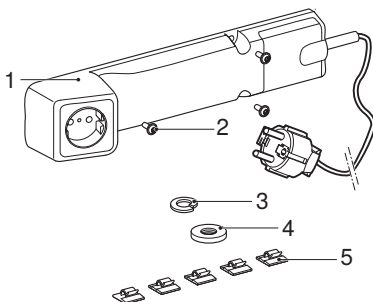
1. Ábra: Geberit aljzatelem
