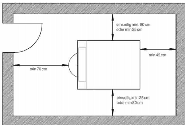
Abb. 1: Empfohlene Wandabstände
