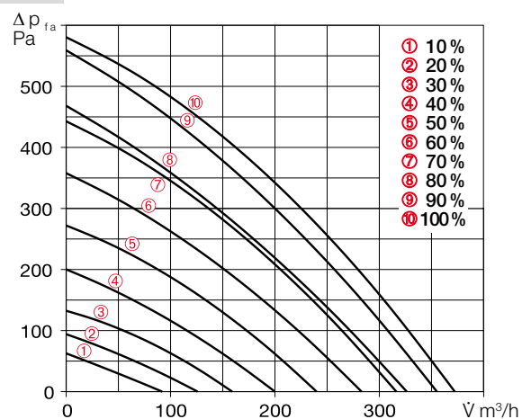
Courbe caractéristique KWL 340 D
