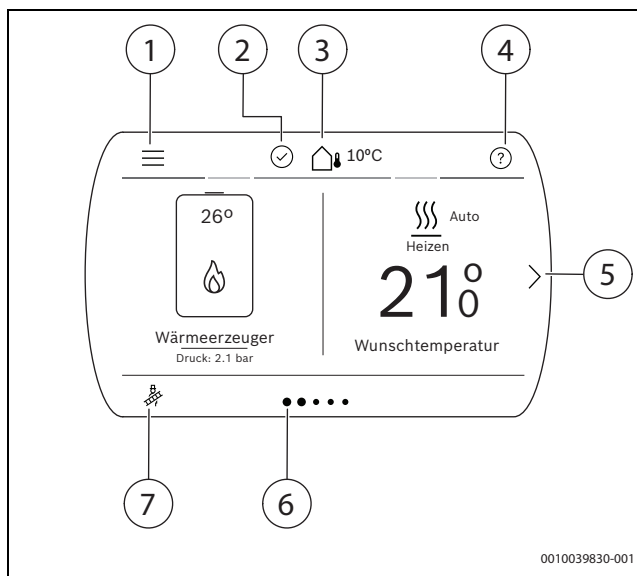
Bild 1 Bedienfeld
