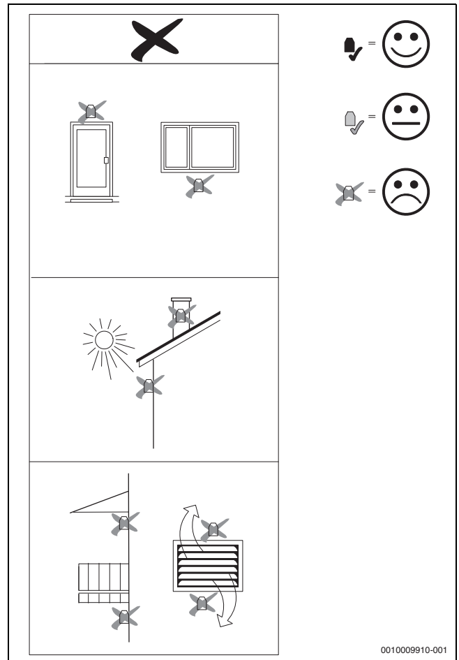
Bild 3 Ungeeigneter Installationsort des Außentemperaturfühlers
