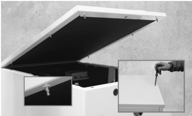
Abb. 57: Demontage der oberen Verkleidung
