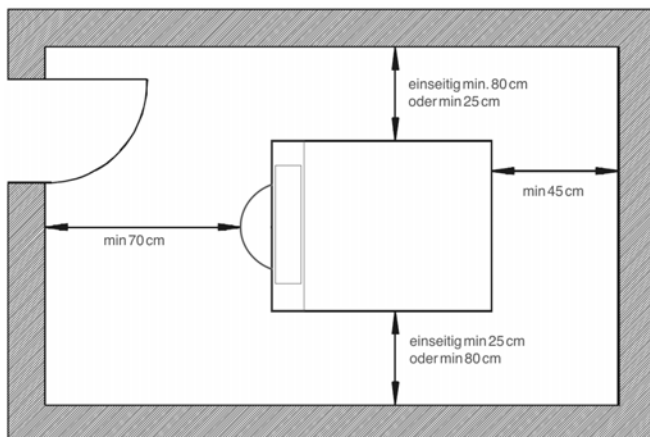
Abb. 1: Empfohlene Wandabstände
