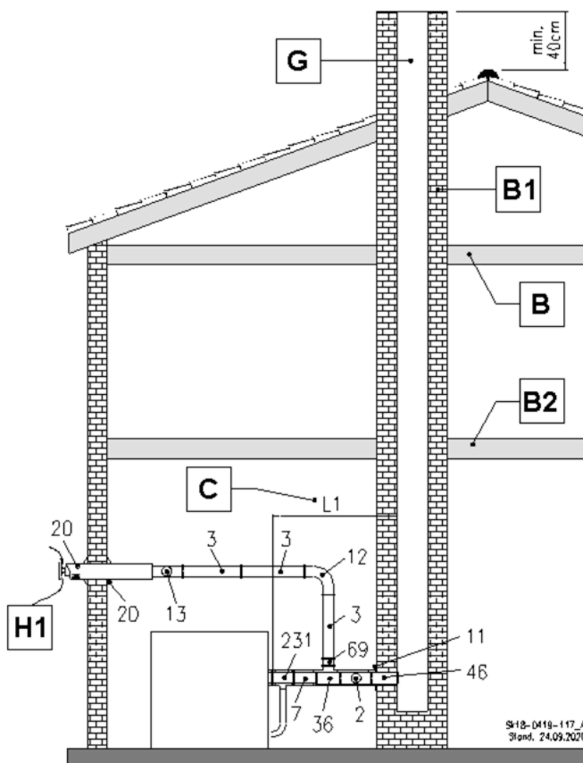
Abb. 35: C 83x Anschluss an einen feuchte-unempfindlichen Abgasschornstein und Zuluft durch die Außenwand
