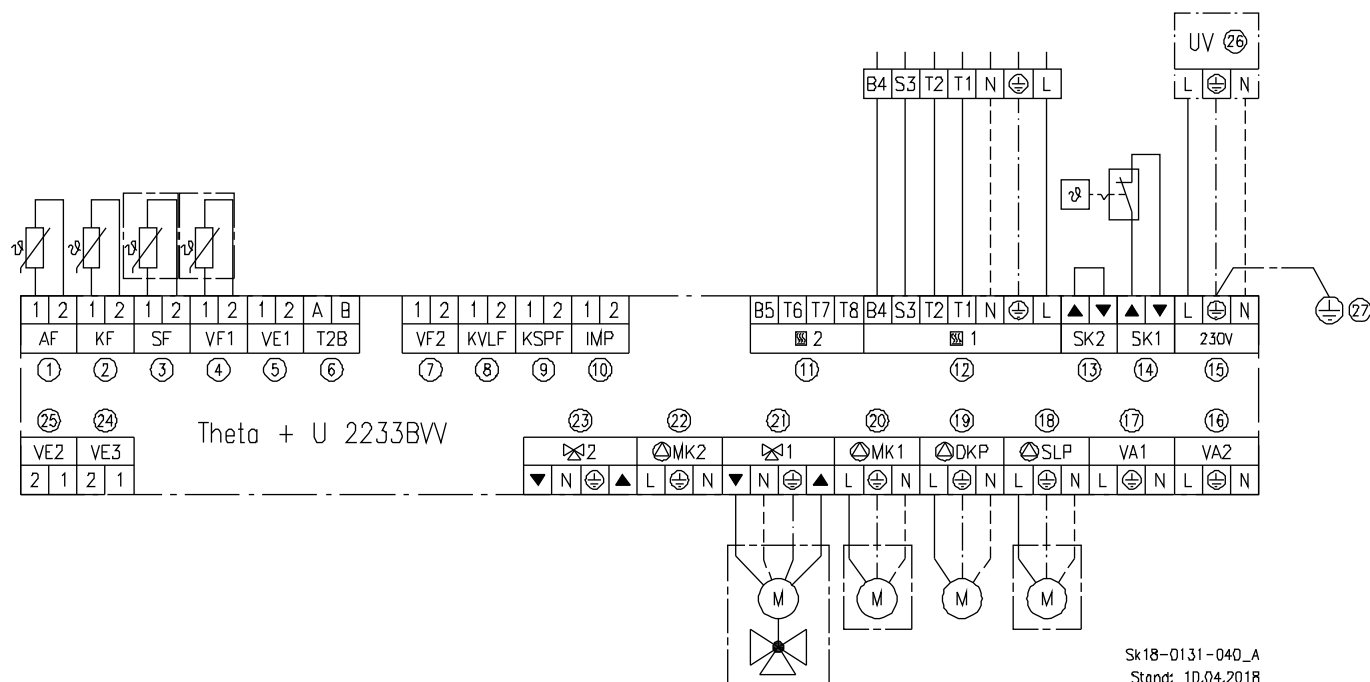
Abb. 25: Elektrische Anschlüsse und Stromlaufplan für ecoDUO... und ecoOEL Pro... (mit Raketenbrenner® RE .. HUG) sowie ecoDUO GAS... (mit Gas-Gebläsebrenner GE..HU)
