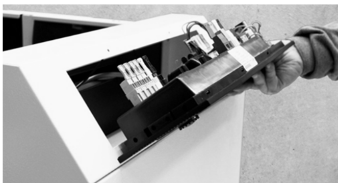
Abb. 18: Ausgeklapptes Unit-Schaltfeld
