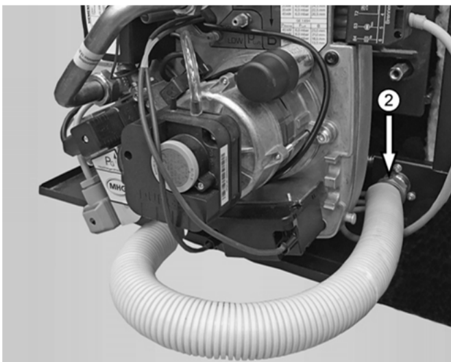
Abb. 11: Brenner-Gasanschluss ② am Kessel
