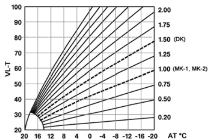
Abb. 56: Heizkennlinie (Steilheit)
