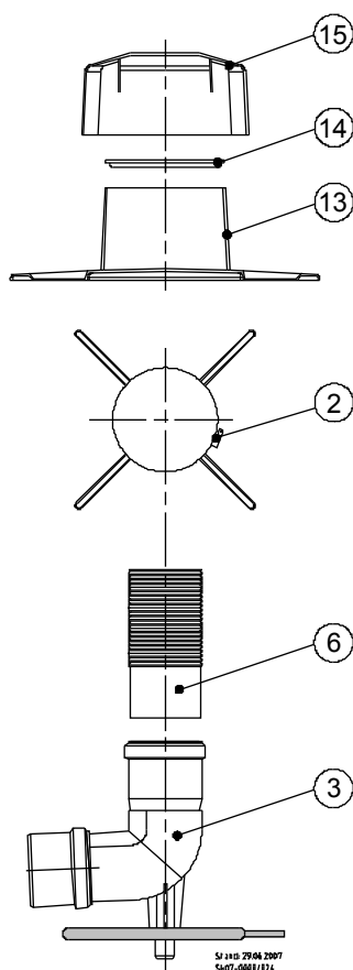
Abb. 46: Detail-Zeichnung Befestigung Schachtabdeckung
