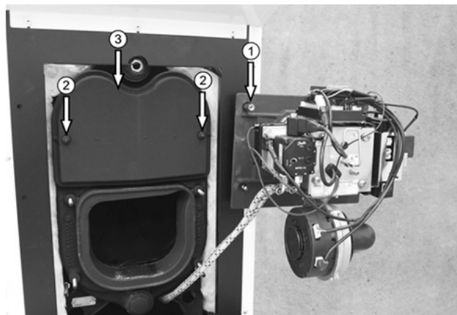
Abb. 64: Brenner-Serviceposition und Demontage der oberen Kesseltür (Der abgebildete Brenner entspricht evtl. nicht dem gelieferten.)
