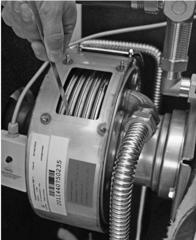
Abb. 70: Anwendung der Reinigungsklinge
