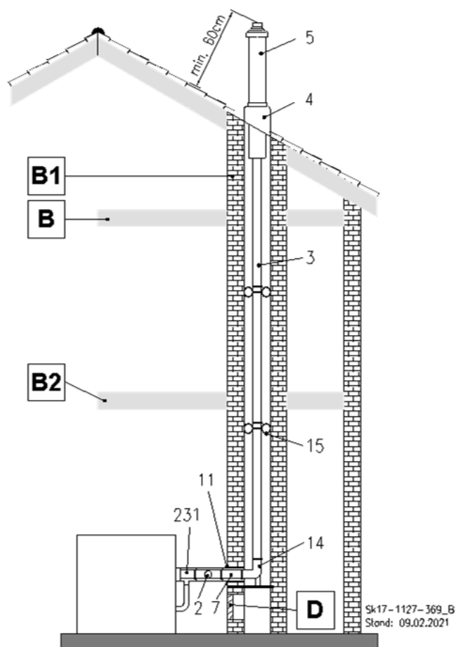
Abb. 36: C 93x Luft-Abgas-System im Schacht und Luft-Abgas-Rohrsystem mit Dachdurchführung
