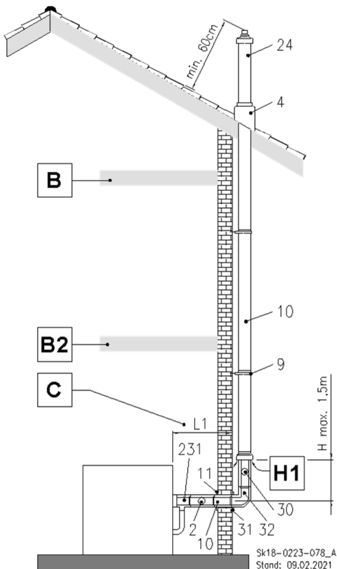
Abb. 33: C 53x Außenwandführung LAS
