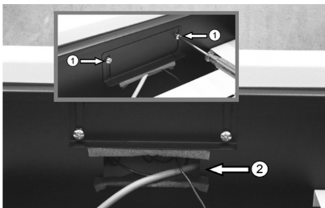
Abb. 19: Kabeldurchführung ② am Schaltfeldgehäuse
