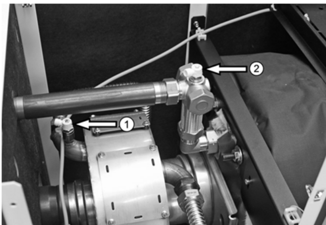
Abb. 16: Kesselkörper-Entlüfter ① sowie RWT-Entlüfter ② (bei Variante ohne interne Kreise)
