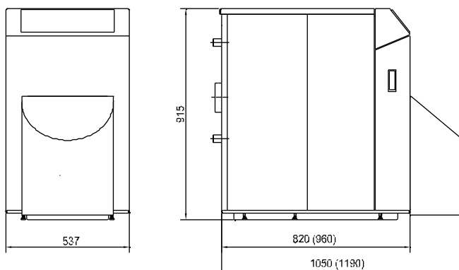
Abb. 2: Abmessungen
