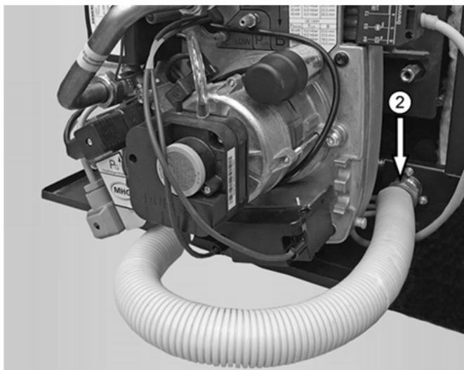
Abb. 62: Brenner-Gasanschluss ② am Kessel
