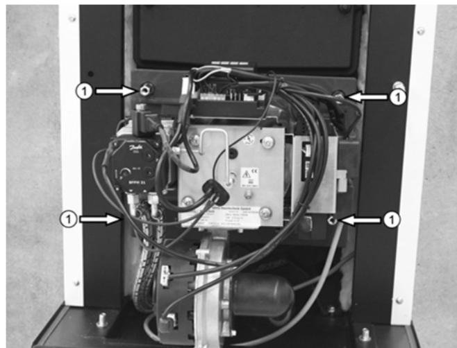
Abb. 63: Muttern ① der unteren Kesseltür (Der abgebildete Brenner entspricht evtl. nicht dem gelieferten.)
