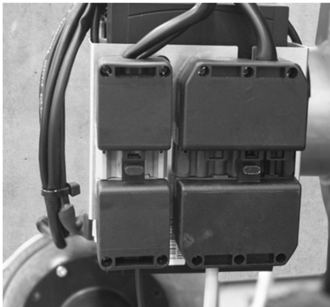
Abb. 61: Euro-Anschluss-Stecker beim RM 1 EUG (Beim RE HU sowie beim GE HU ist der 4-polige Euro-Anschluss-Stecker nicht enthalten.)
