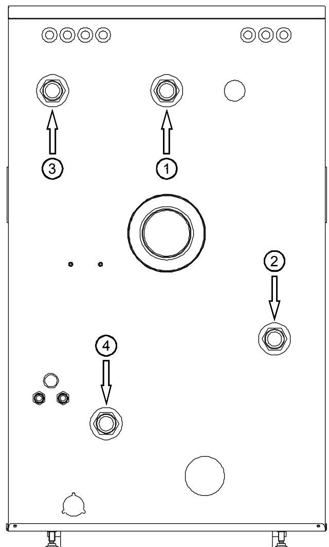
Abb. 12: Hydraulische Anschlüsse an der Kesselrückwand
