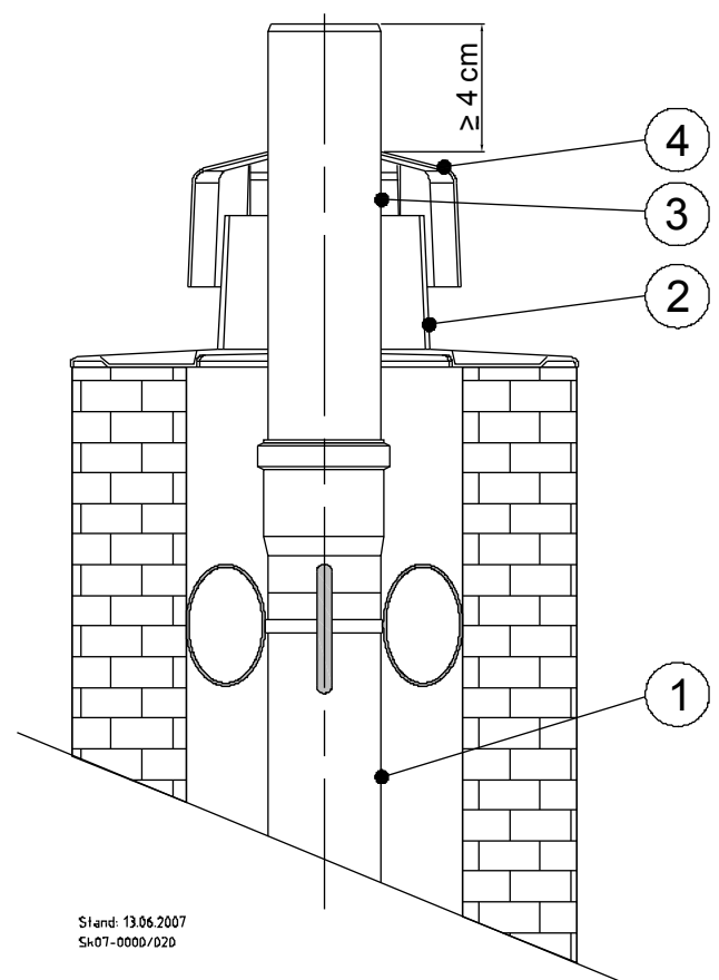
Abb. 42: Schachtabdeckung
