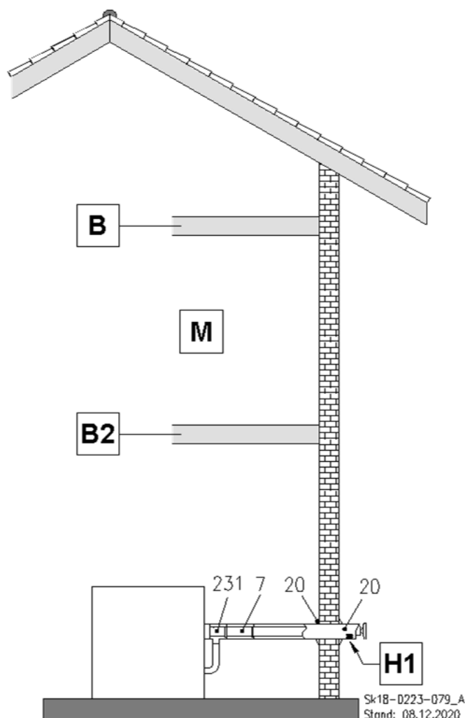
Abb. 30: C 13x Luft-Abgas-Rohrsystem horizontal durch die Außenwand
