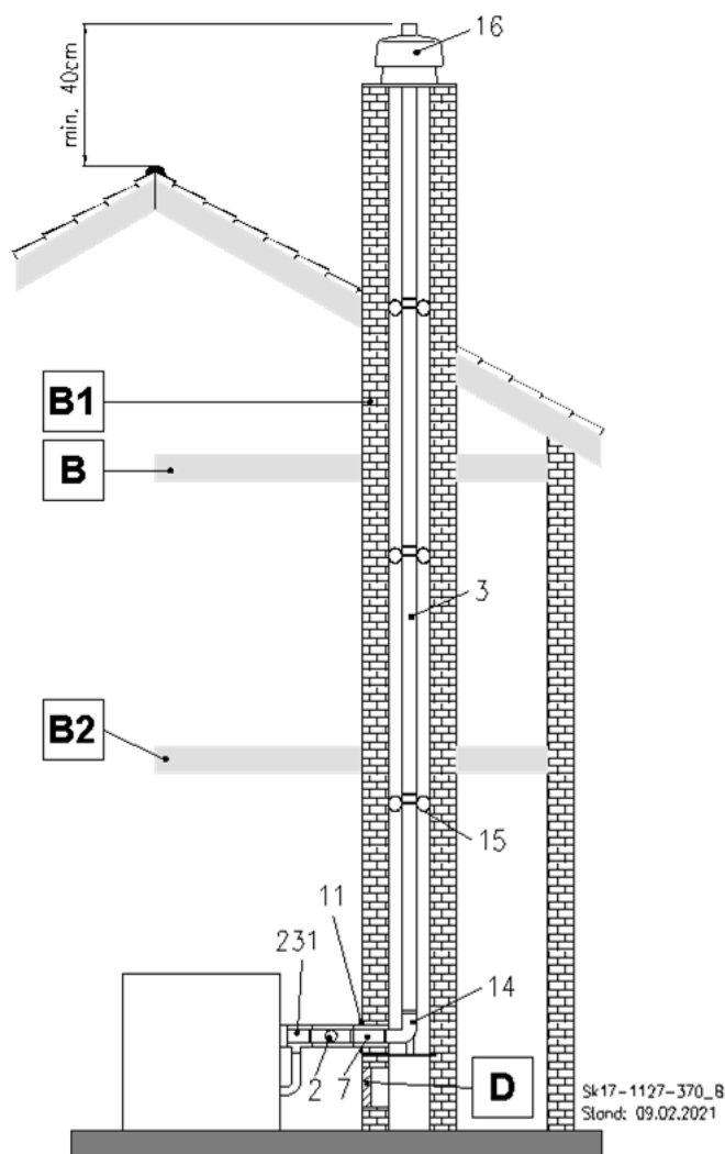
Abb. 37: C 93x Abgasrohr im Schacht
