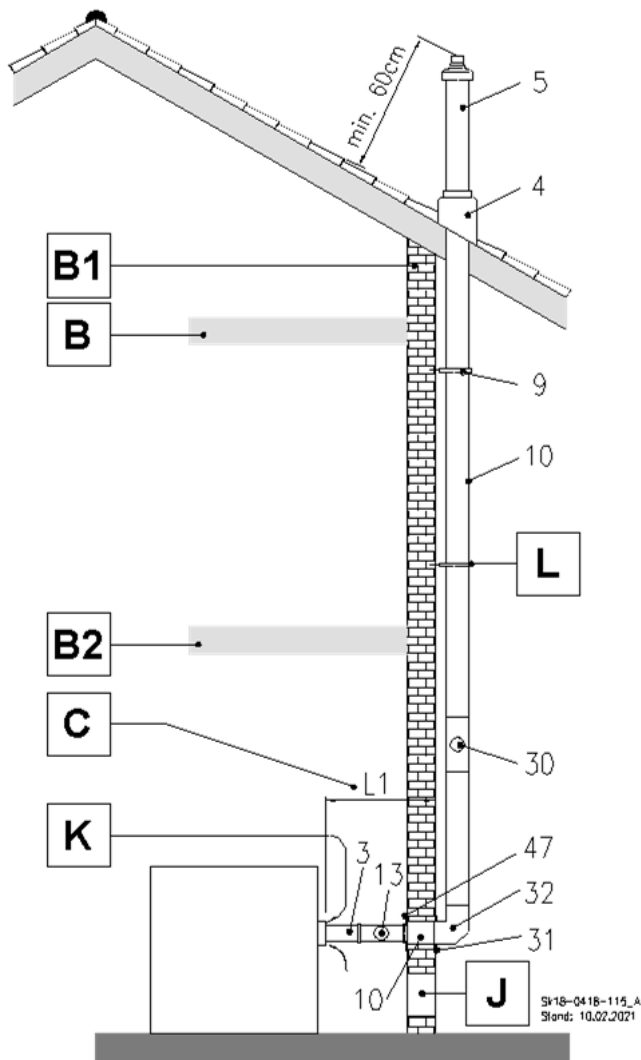
Abb. 27: B 23 Abgasrohr an der Außenwand
