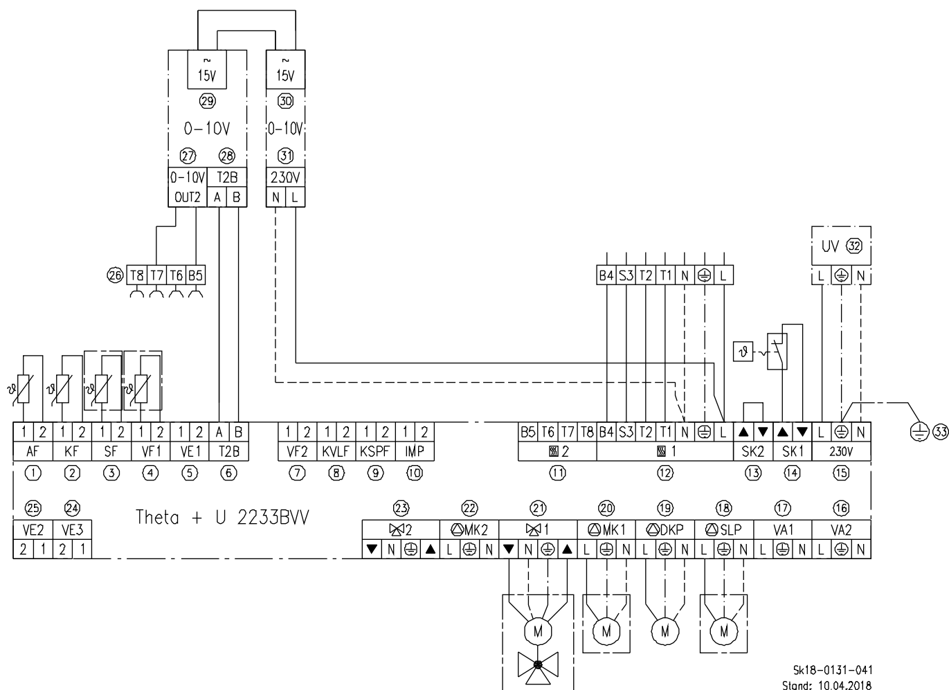
Abb. 24: Elektrische Anschlüsse und Stromlaufplan für ecoDUO...m (Raketenbrenner® RM .. EUG)
