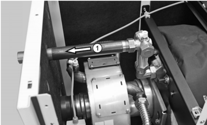
Abb. 13: Vorlauf Direktkreis ① (bei Standardausführung ecoDUO .. / ecoOEL Pro ..)
