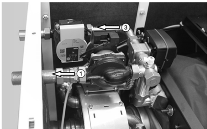
Abb. 14: Vorlauf Direktkreis ① sowie Vorlauf Mischer- kreis ③ (bei Ausführung ecoDUO ..i)
