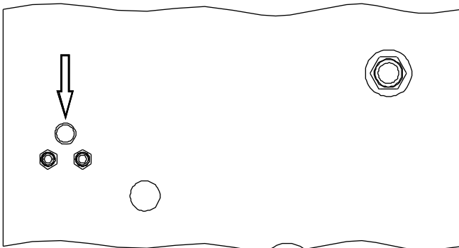
Abb. 7: Kondensatablauf
