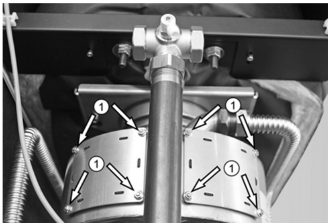
Abb. 67: Befestigungsmuttern ① der Reinigungsabdeckungen vom RWT
