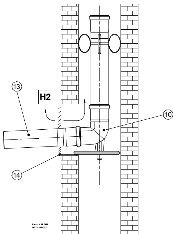
Abb. 43: Schachteinführung
