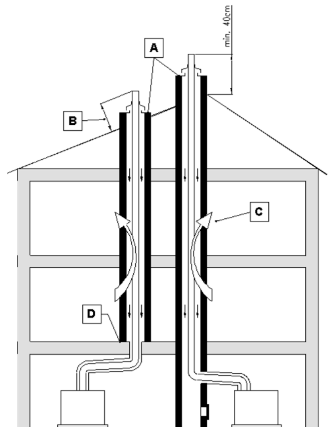
Abb. 26: Schachtqualität für Abgasleitungen
