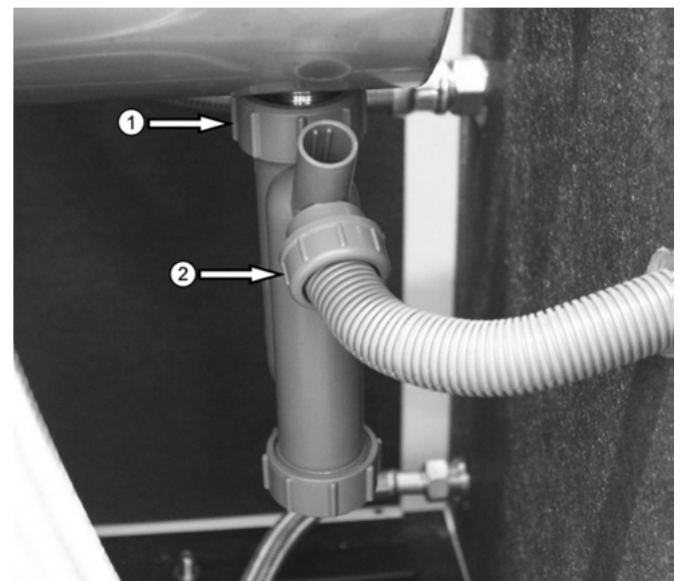
Abb. 66: Demontage des Kondensat-Siphons
