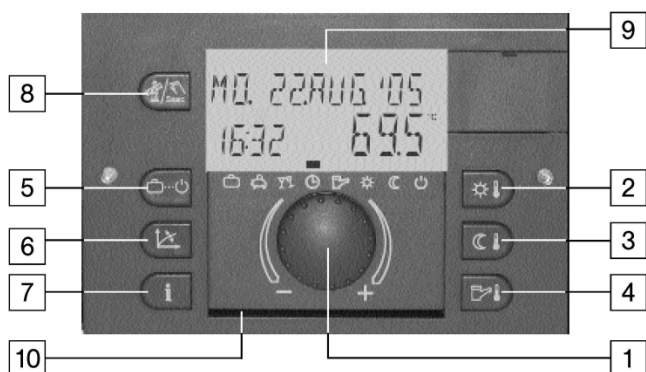
Abb. 55: Bedieneinheit
