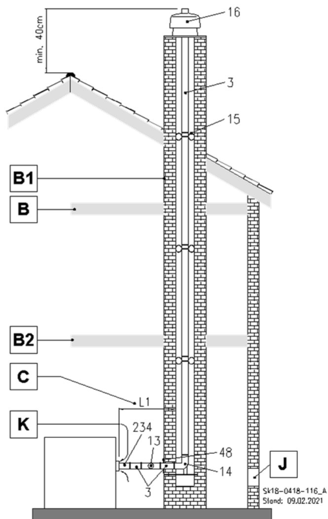
Abb. 28: B 23 Abgasrohr im Schornstein
