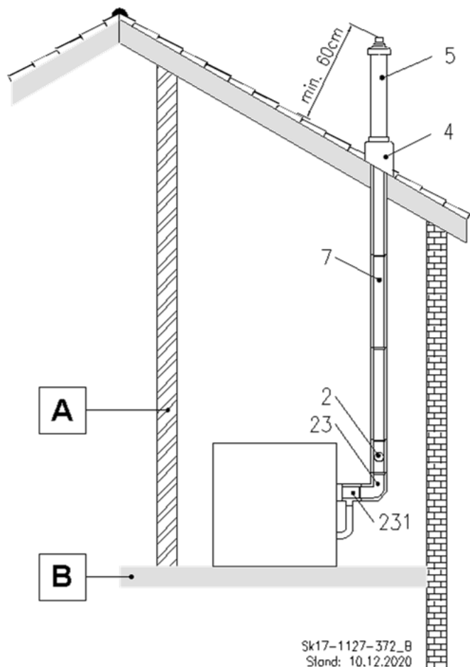
Abb. 32: C 33x Dachheizzentrale mit der Durchführung senkrecht durch ein Schrägdach
