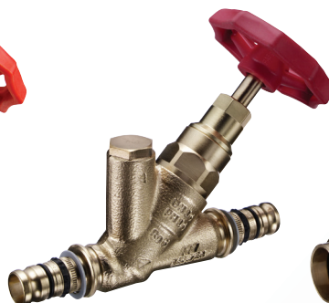
WESER Freistrom-Absperrventil, mit Entleerstopfen, mit fest inte- griertem Pressanschluss auf MEPLA, Figur 190 40
