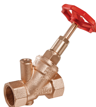
WESER Freistrom-Absperrventil, mit Entleerstopfen, IG, Figur 190 02
