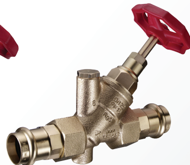
WESER Freistrom-Absperrventil, mit Entleerstopfen, mit fest inte- griertem Pressanschluss auf SANPRESS/PROFIPRESS, Figur 190 30
