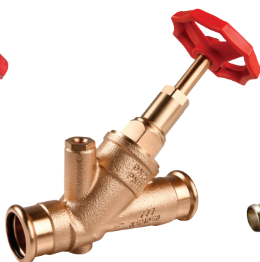
WESER Freistrom-Absperrventil, mit Entleerstopfen, mit fest inte- griertem Pressanschluss auf MAPRESS, Figur 190 22
