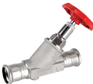
NIRO Freistrom-Absperrventil, ohne Entleerung, mit fest integriertem Pressanschluss auf MAPRESS, Figur 073 00
