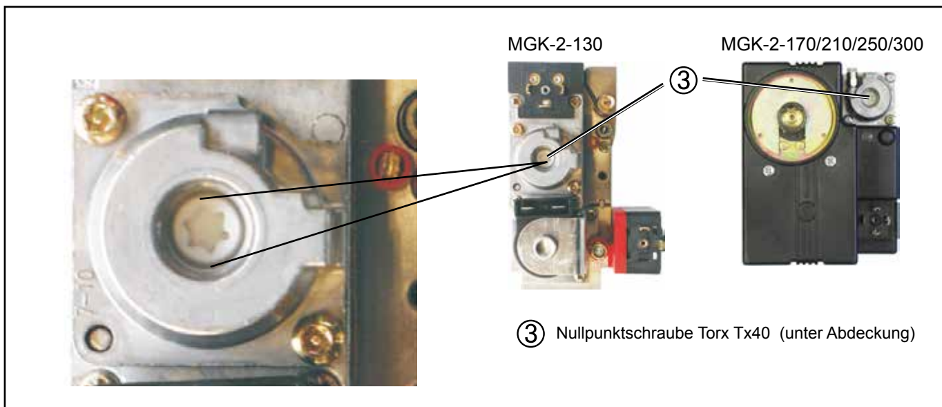
Bild: Gaskombiventil
