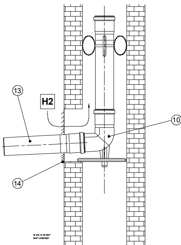
Abb. 43: Schachteinführung
