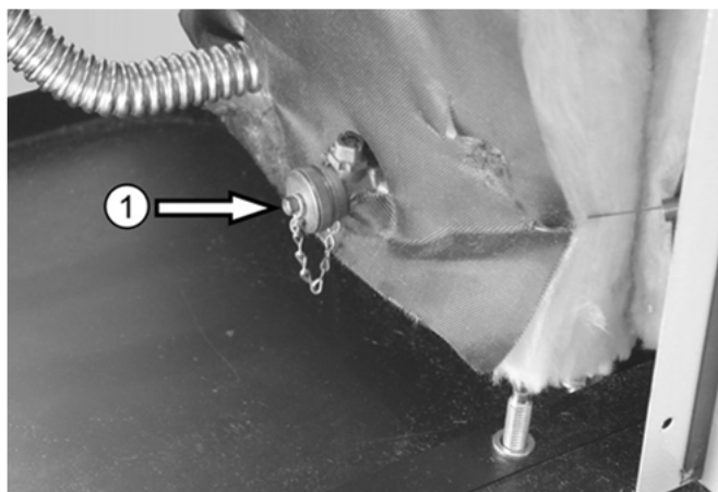
Abb. 15: Kesselfüll- und Entleerhahn ①
