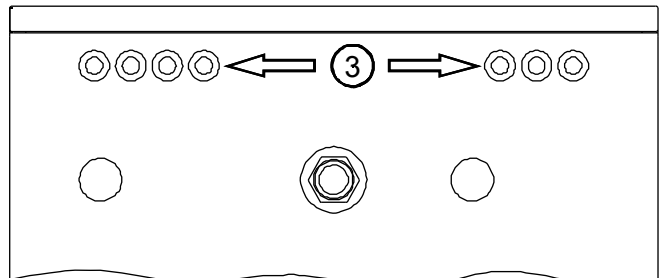
Abb. 20: Kabeldurchführungen ③ in der Rückwand
