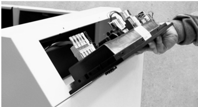
Abb. 18: Ausgeklapptes Unit-Schaltfeld
