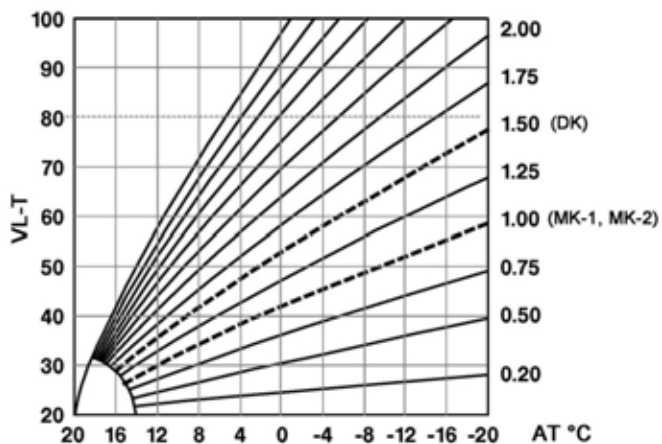
Abb. 56: Heizkennlinie (Steilheit)
