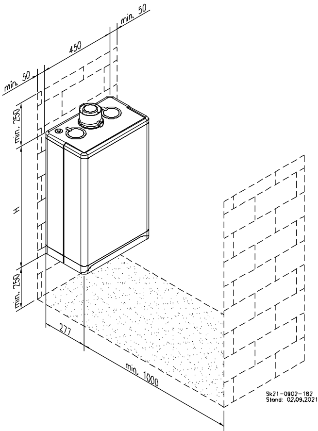
Abb. 3: Montageabstände
