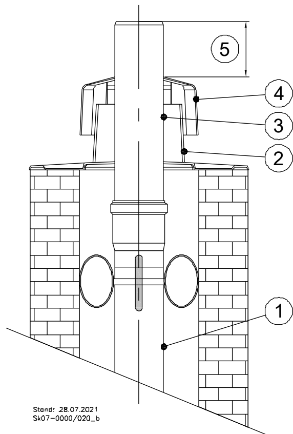
Abb. 58: Schachtabdeckung
