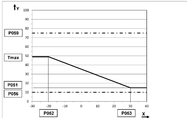
Abb. 88: Heizkennlinie mit geänderten Einstellungen
