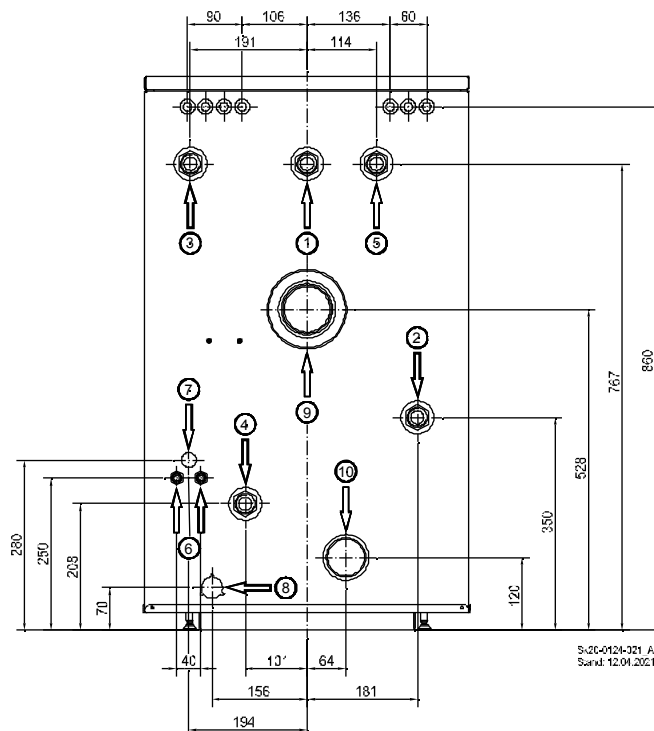
Abb. 3: Abmessungen Rückseite
