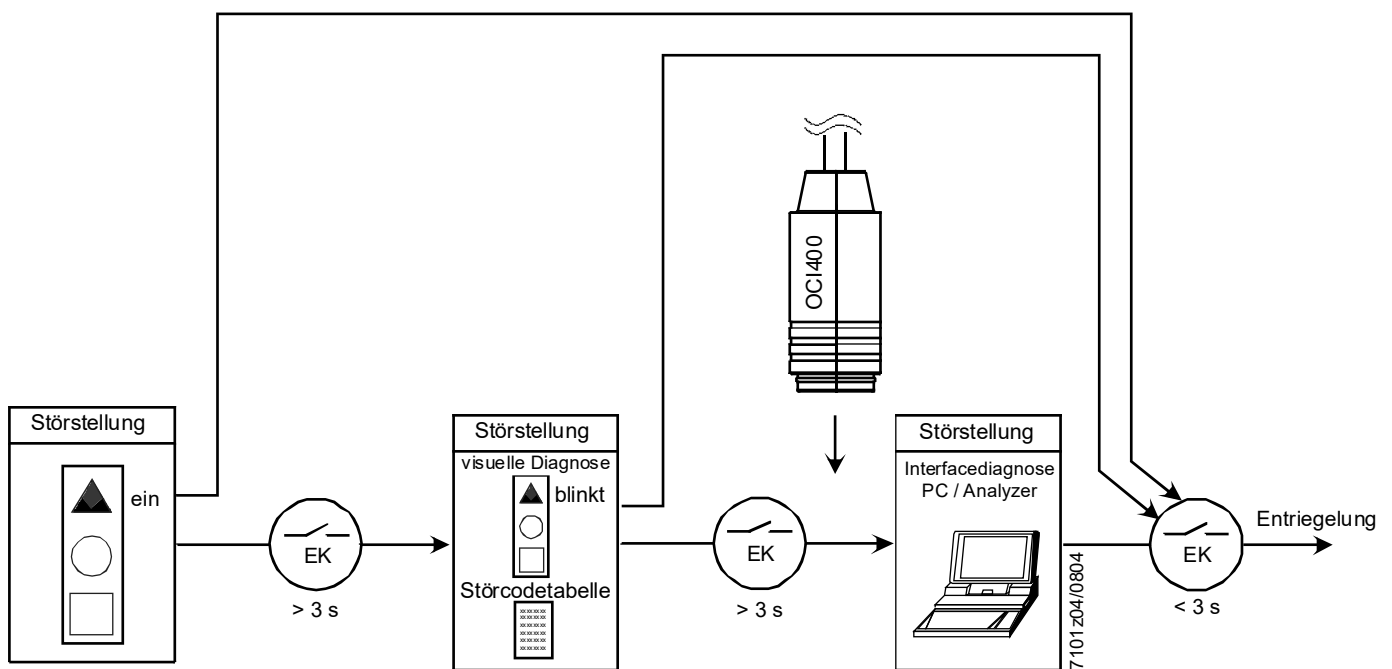
Abb. 43: Ablauf Störursachendiagnose
