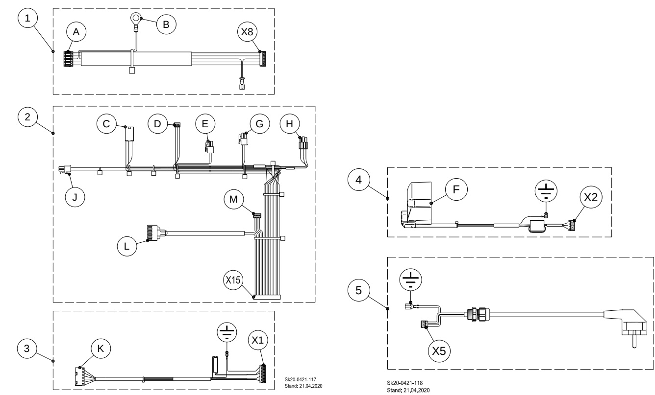
Abb. 98: Verdrahtung
