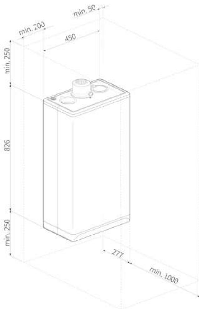
Abb. 3: Montageabstände
