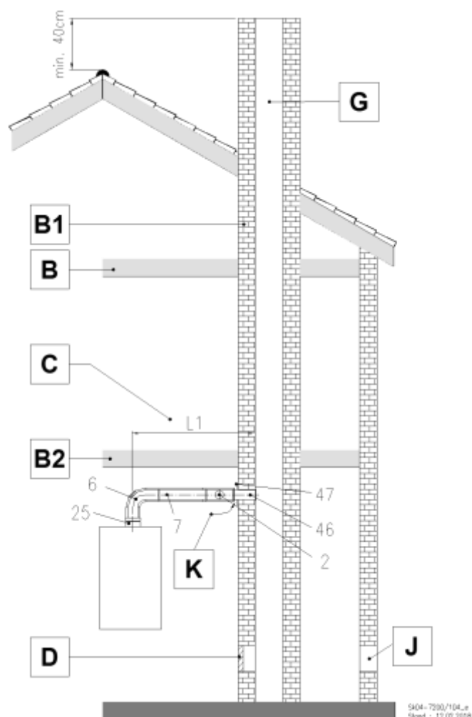
Abb. 29: B 33 Abgasrohr endet im feuchteunempfindlichen Schornstein
