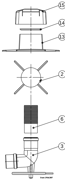
Abb. 47: Detail-Zeichnung Befestigung Schachtabdeckung
