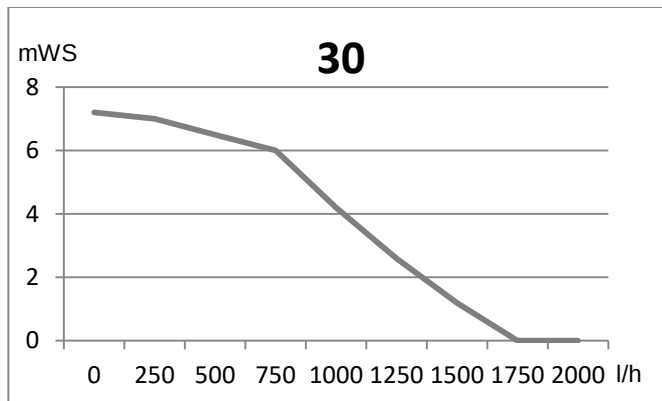
Abb. 103: Restförderhöhe ecoGAS Pro 30, ProX 30/38
