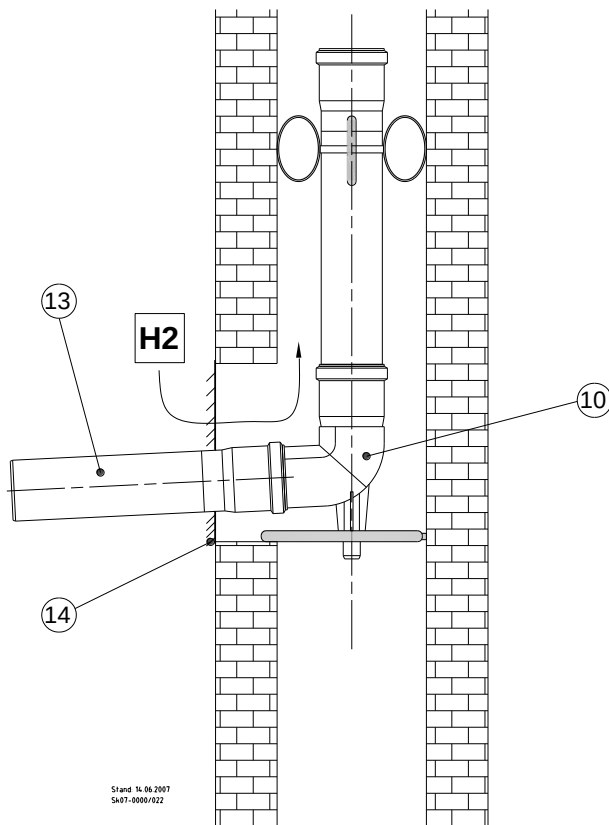
Abb. 44: Schachteinführung
