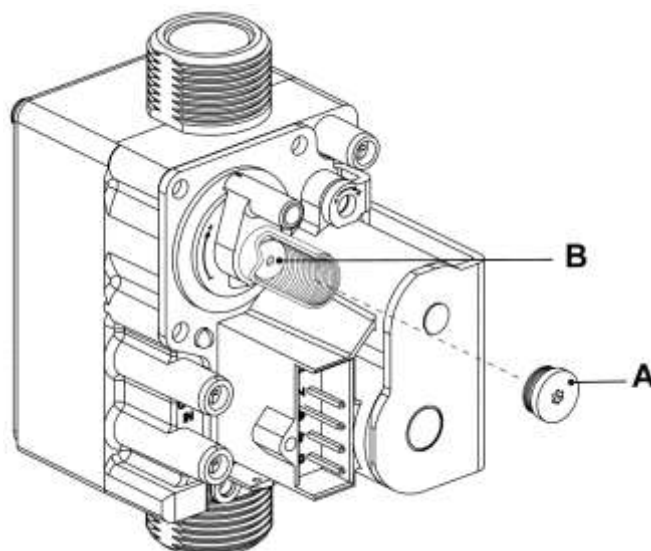
Abb. 77: Gasventil
