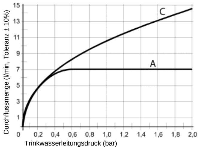
Abb. 13: Widerstandsdiagramm Trinkwasser-Tauscher-schlange
