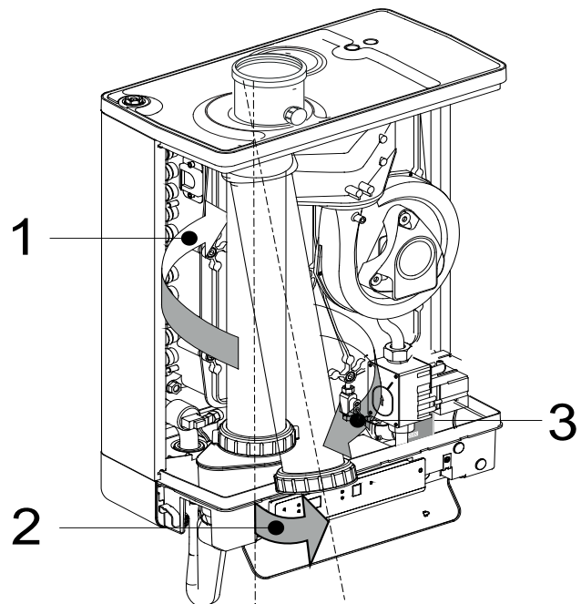
Abb. 79: Demontage Abgasrohr
