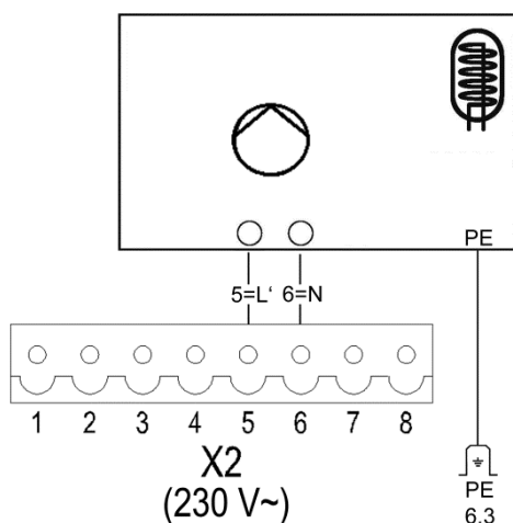
Abb. 28: Anschluss Ladepumpe für Trinkwarmwasserspeicher
