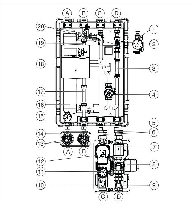
Abb. 2: Aufbau Regudis H-HT
