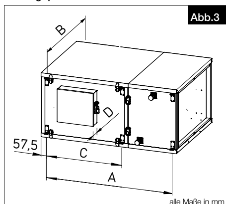
Abhängepunkte
