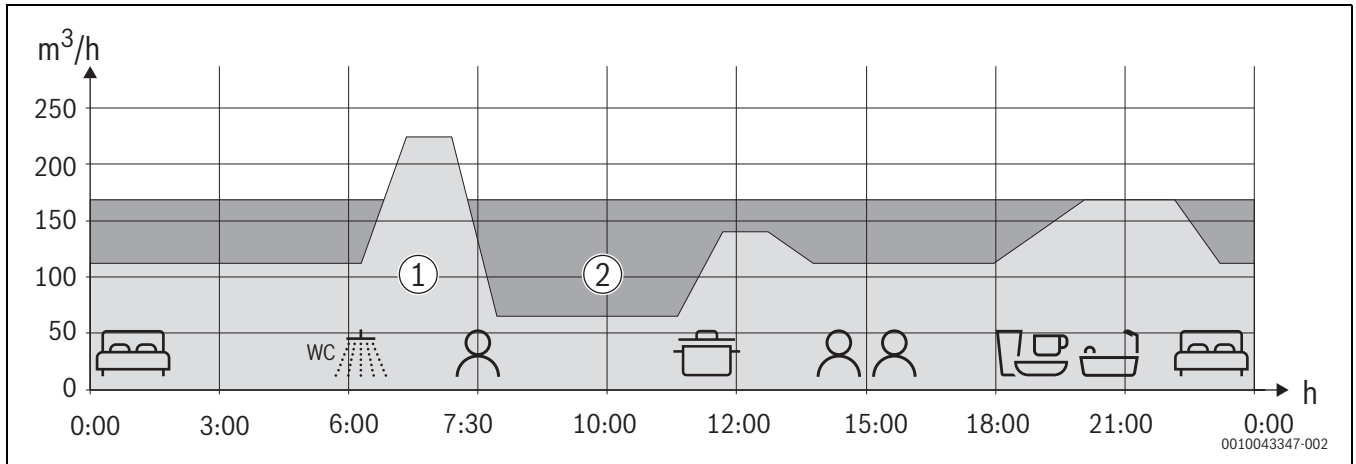
Bild 4 Beispielhafter Vergleich der bedarfsgeregelten/manuellen Lüftung
