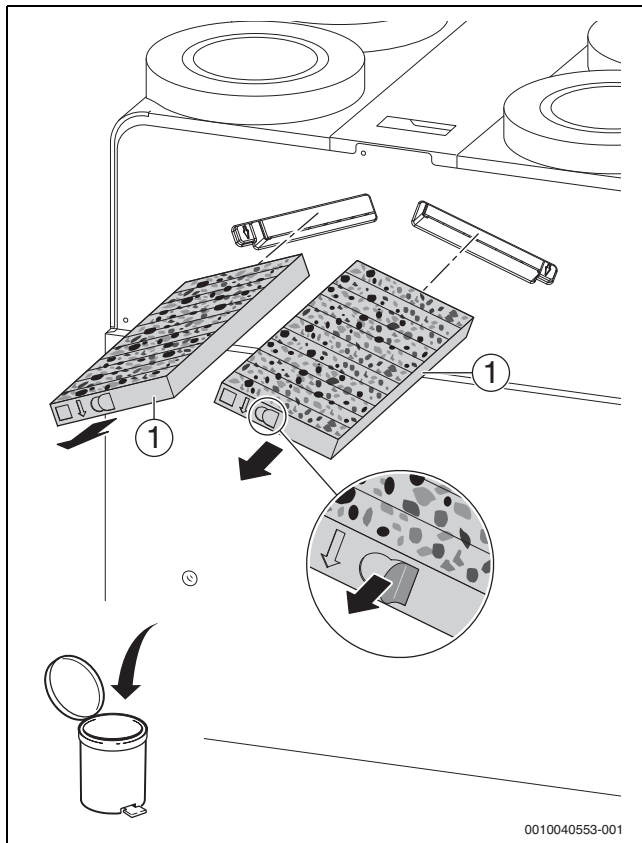
Bild 7 Filter herausziehen
