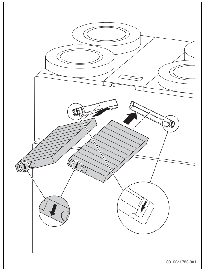
Bild 8 Filter einschieben
