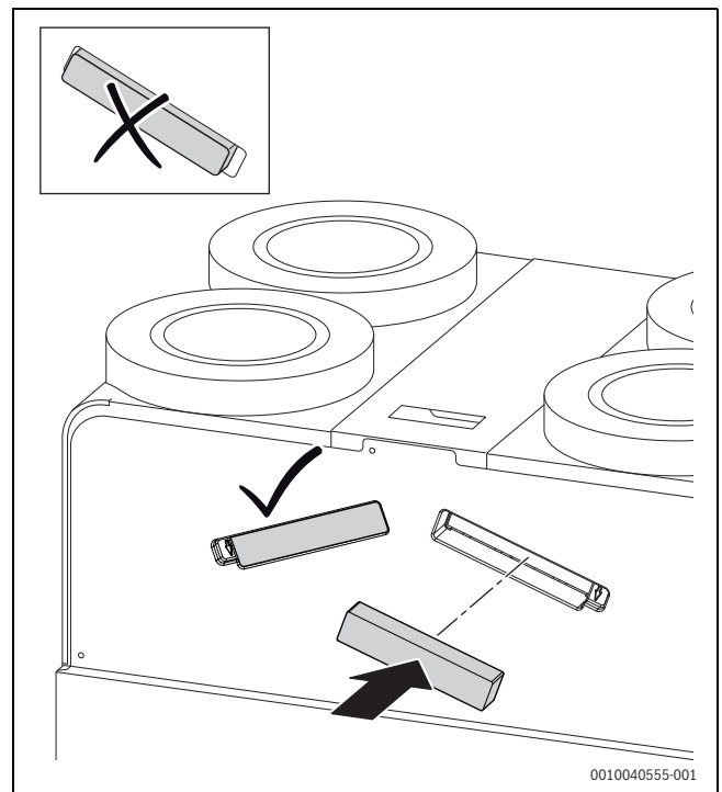
Bild 9 Filterabdeckung montieren
