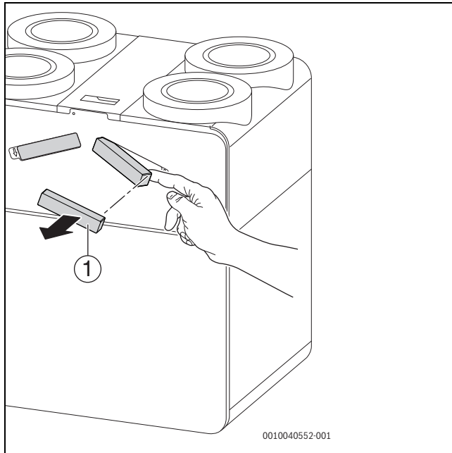
Bild 6 Filter herausziehen
