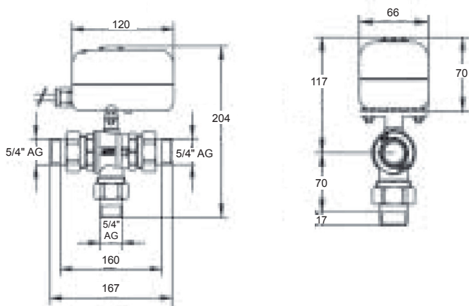
DN 32 • Massangaben in mm
