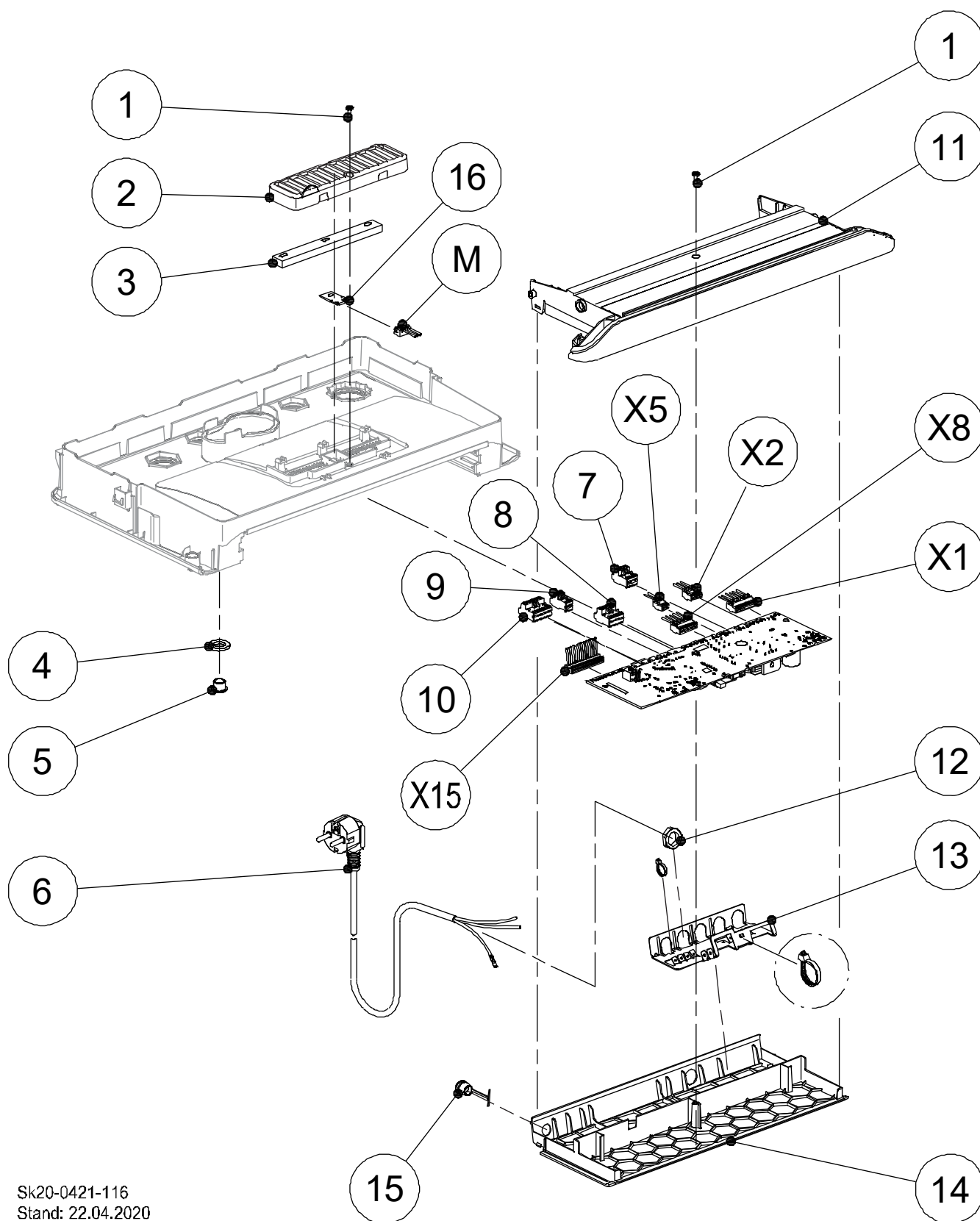
Abb. 115: Regelung und Elektrik
