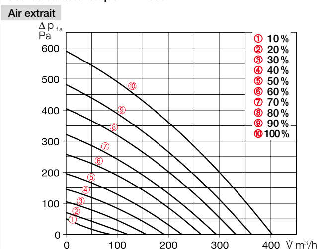
Courbe caractéristique KWL 360 W ET
