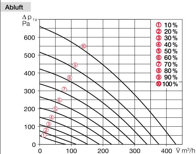
Kennlinie KWL 360 W
