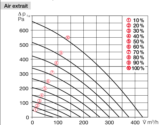
Courbe caractéristique KWL 360 W
