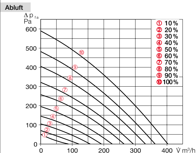
Kennlinie KWL 360 W ET
