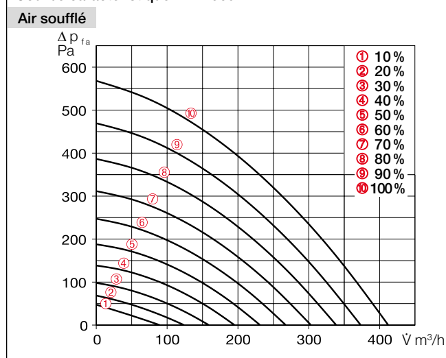
Courbe caractéristique KWL 360 W ET
