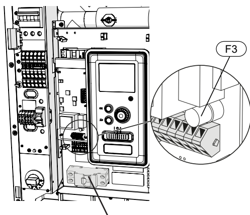
Fehlerschutzschalter RCD
