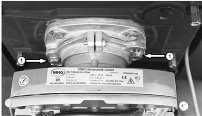
Abb. 30: Brennerbefestigungsschrauben
