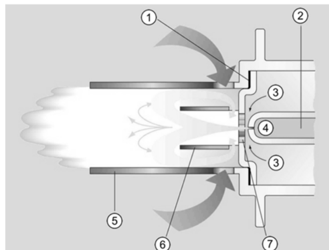
Abb. 47: Verbrennungsablauf Raketenbrenne®
