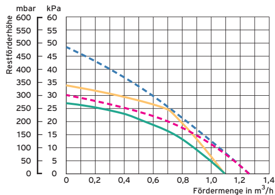
Pumpendiagramm VCC 266/4-5
