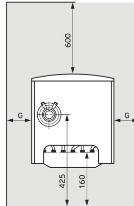
Draufsicht
