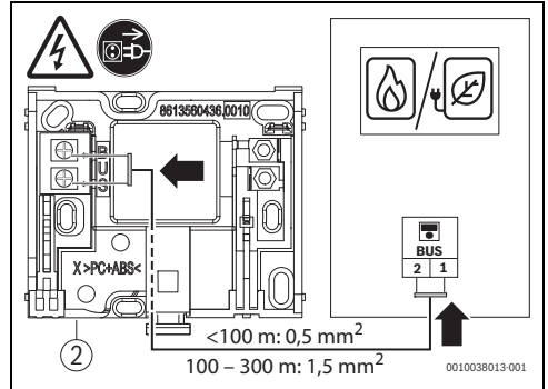
Bild 6 Anschluss der Bedieneinheit an einem Wärmeerzeuger
