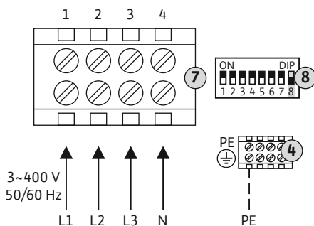
Fig. 7: Netzanschluss 3~400 V ohne Hauptschalter
