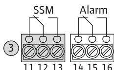
Fig. 14: Klemmleiste Sensorik: SSM
