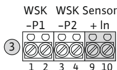
Fig. 12: Klemmleiste Sensorik: Anschluss Niveaueinfassung
