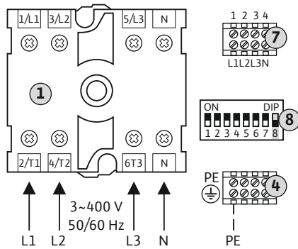
Fig. 5: Netzanschluss 3~400 V mit Hauptschalter
