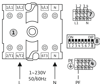
Fig. 4: Netzanschluss 1~230 V mit Hauptschalter
