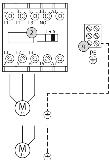
Fig. 8: Pumpenanschluss
