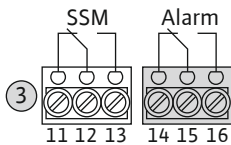
Fig. 15: Klemmleiste Sensorik: externer Alarmmelder für Hochwasser
