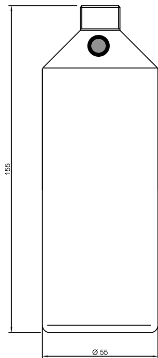
Behälter MF050 250ml Art. Nr. 14635400
