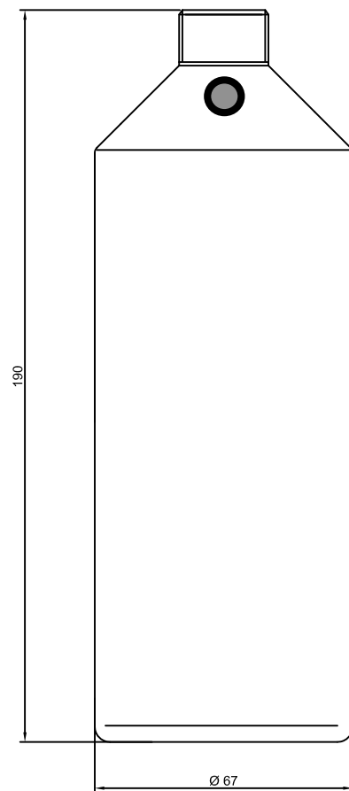
Behälter MF050 500ml Art. Nr. 14635411
