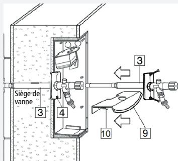
Montage en surface
