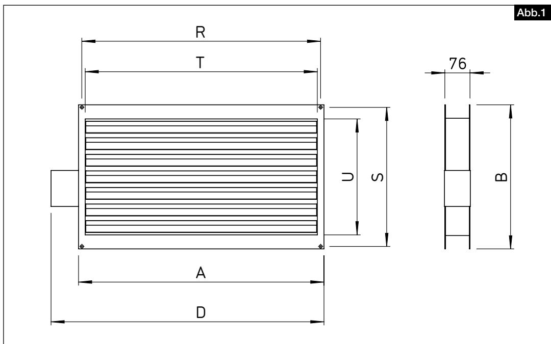
Abmessungen Jalousie-Verschlussklappe für AIR1 XC/XVP Geräte
