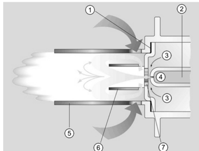
Abb. 47: Verbrennungsablauf Raketenbrenne®
