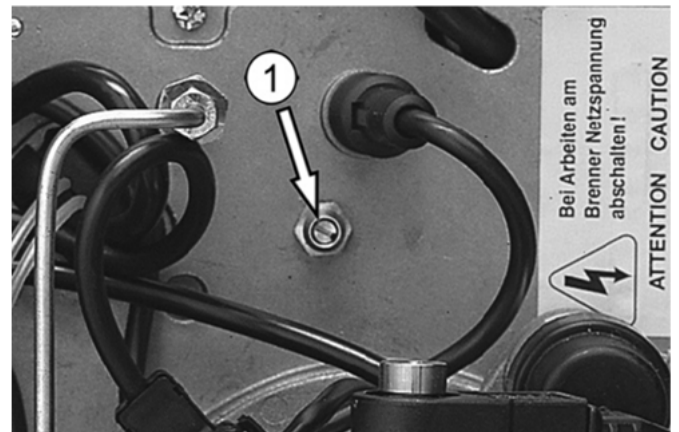
Abb. 23: Messnippel ① zur Prüfung der Gebläsepression
