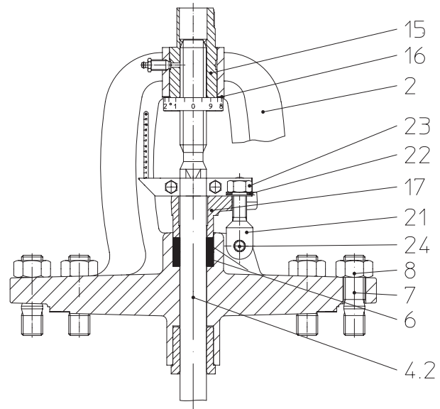
Bild 8: DN250-400
