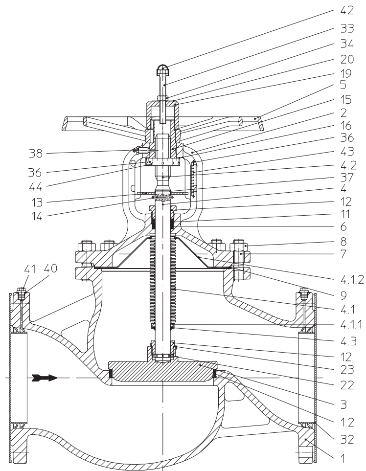
Bild 4: DN 200 mit Hubskala
