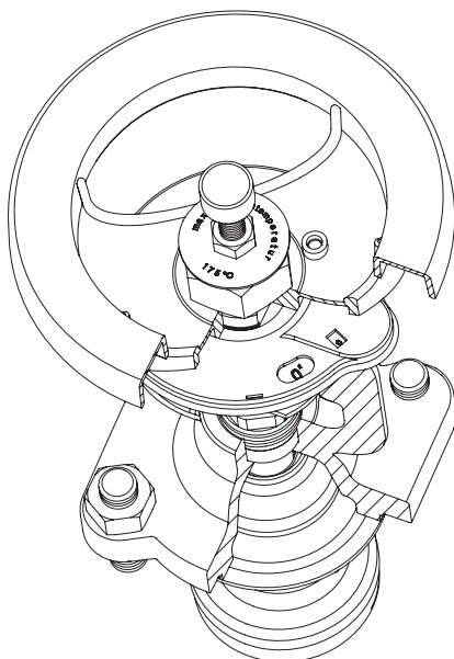
Bild 1: DN 15- 150 mit digitaler Anzeige
