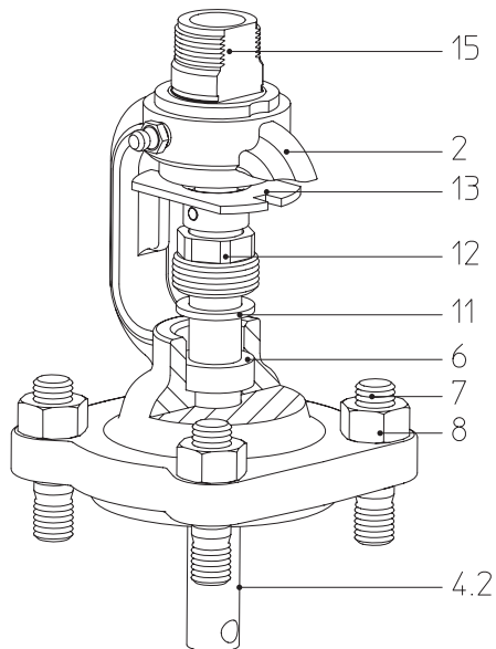
Bild 7: DN15-200
