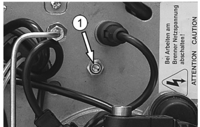
Abb. 23: Messnippel ① zur Prüfung der Gebläsepression
