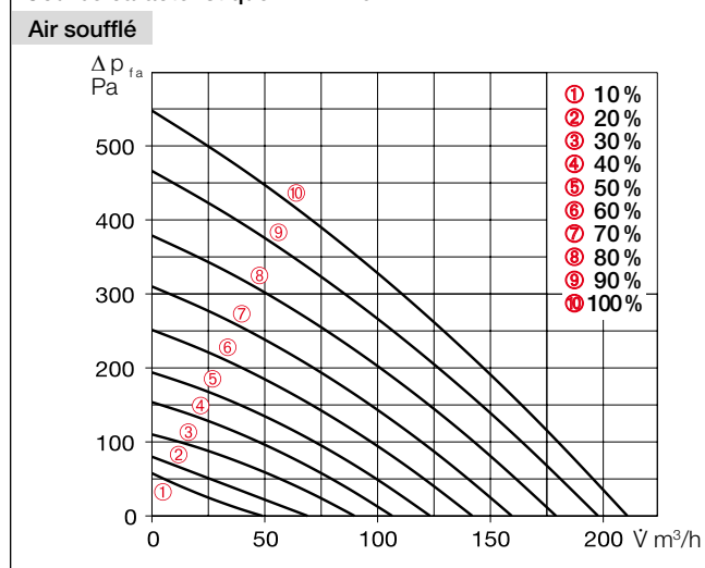
Courbe caractéristique KWL 170 W ET
