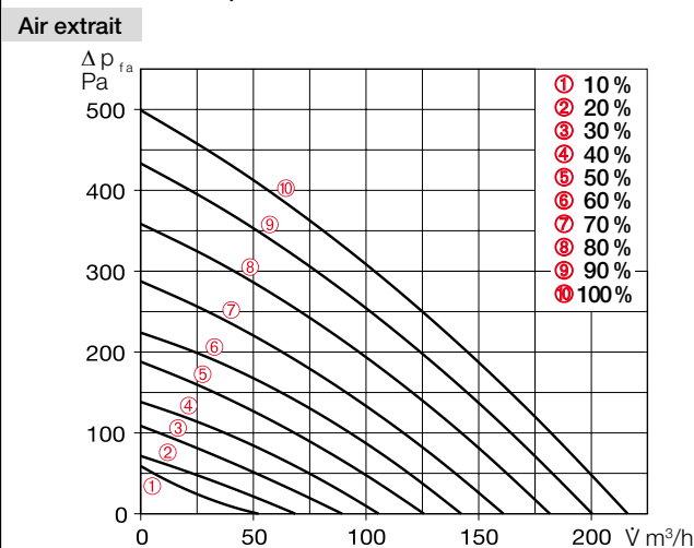
Courbe caractéristique KWL 170 W
