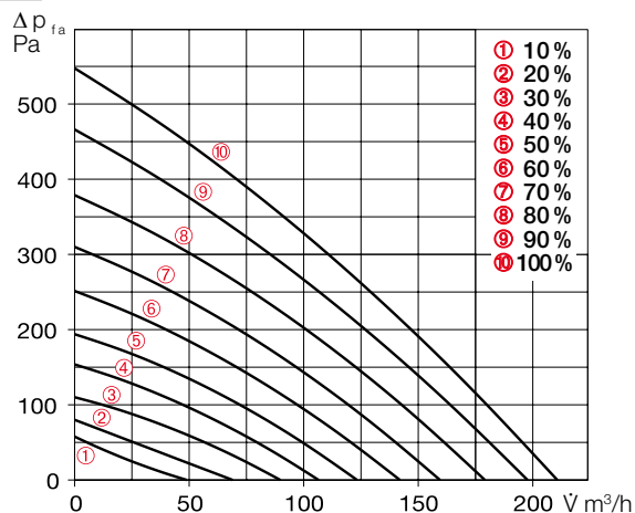
Kennlinie KWL 170 W ET
