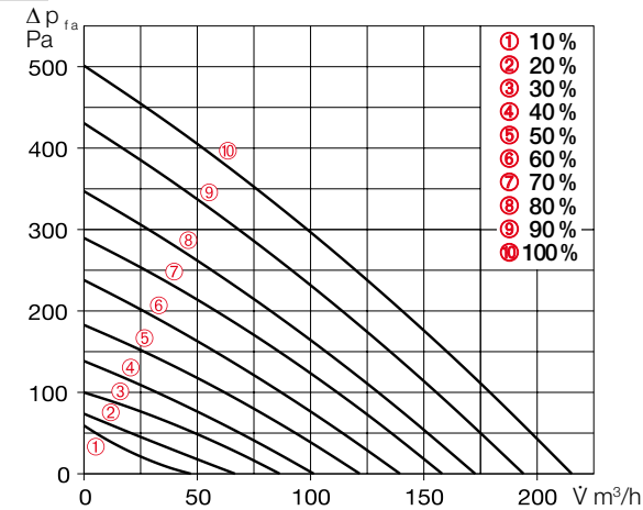
Kennlinie KWL 170 W ET
