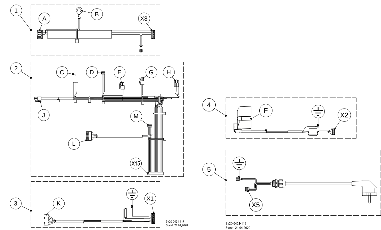
Abb. 98: Verdrahtung
