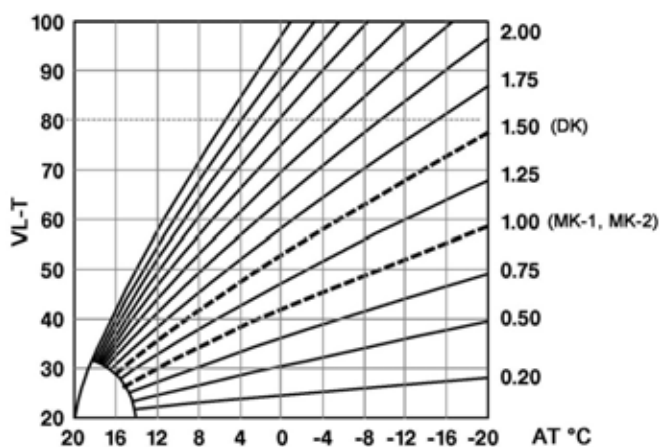
Abb. 56: Heizkennlinie (Steilheit)
