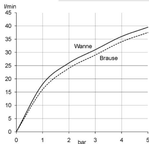
Durchflussdiagramm
