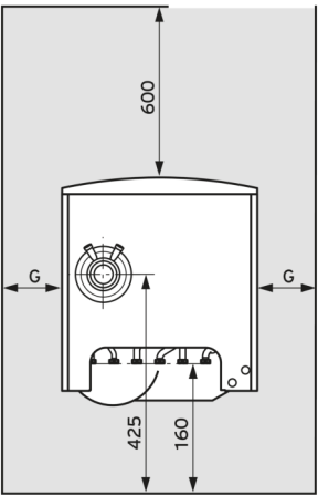
Draufsicht
