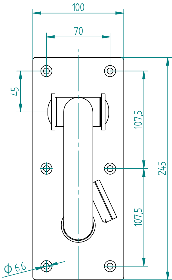
Montageskizze & Bohrbild
