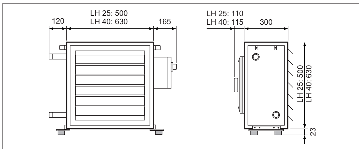
Abb. 11.1 Abmessungen
