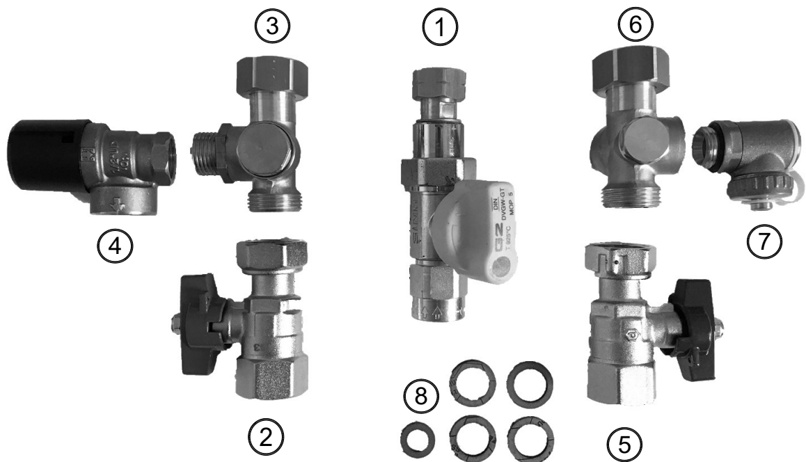
Abb./Fig. 1: Lieferumfang Anschluss-Set Heizer 96.33000-7225
