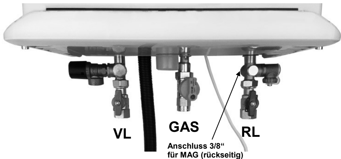
Abb. 2: Hydraulische Heizkreisanschlüsse inkl. Sicherheitsventil, Gaskugelhahn sowie KFE-Hahn
