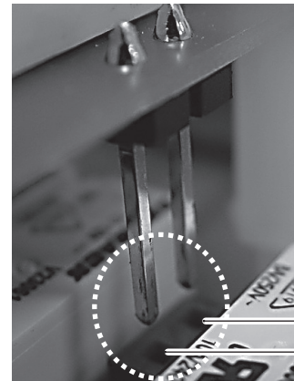
Buchse für 2 obere Kontaktstifte der Comfort-Platine 2.0
