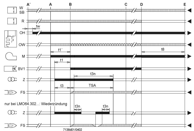
Abb. 33: Programmablauf LMO 64.301 mit Nachlüftungsfunktion (RE 1 HG)
