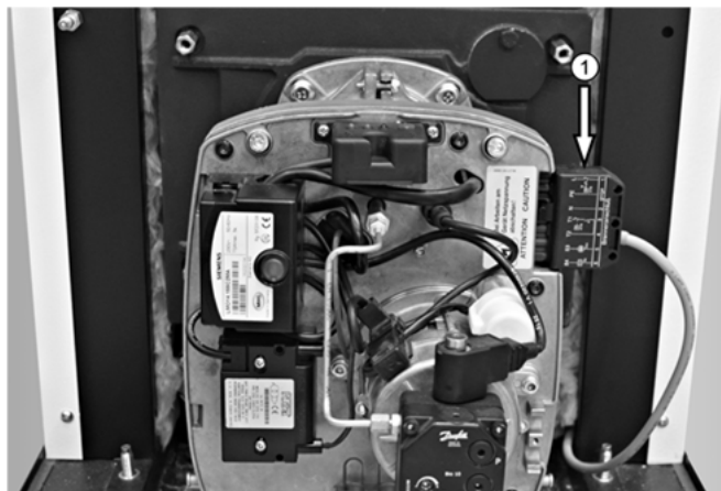
Abb. 12: Montage des Euro-Anschluss-Steckers ①
